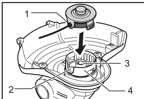
► 1. Ojal del cordón de nailon 2. Muesca del puerto de instalación de la cabeza cortadora de nailon 3. Resorte 4. Sujetador del carrete
